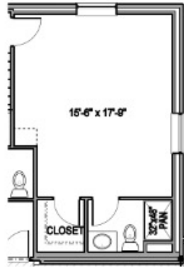
OPT. BEDROOM 4
